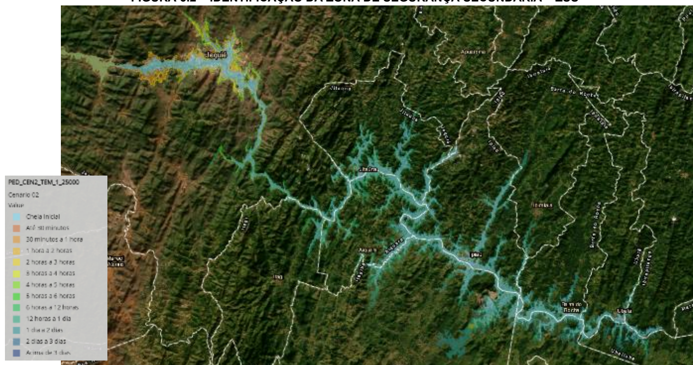
FIGURA 6.2 – IDENTIFICAÇÃO DA ZONA DE SEGURANÇA SECUNDÁRIA – ZSS
